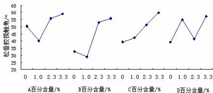
图 2-1 松香胶接触角
